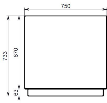
Planter mod. QUADRA H700
