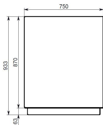
Planter mod. QUADRA H900
